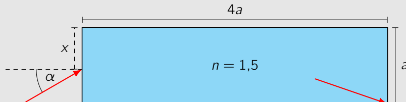
Abb. 13. Nicht maßstabsgetreue Skizze des Laserstrahls im Glasquader in der Seitenansicht.
