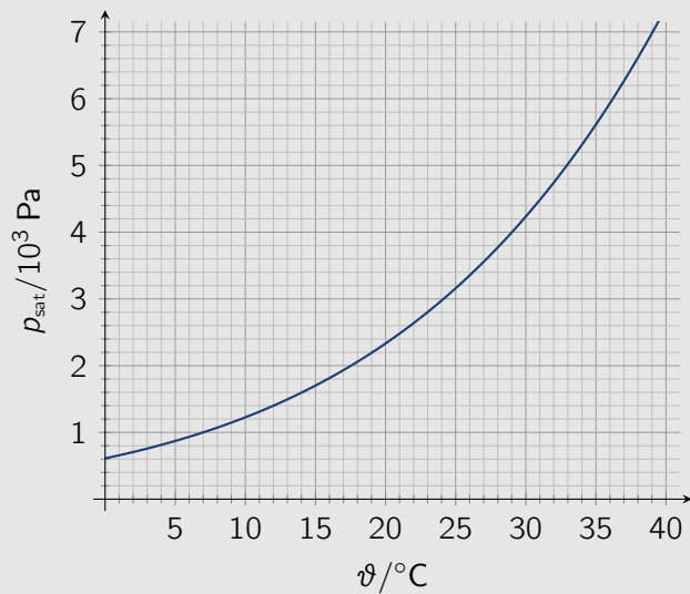
Abb. 12. Sättigungsdampfdruckkurve für Wasserdampf.
