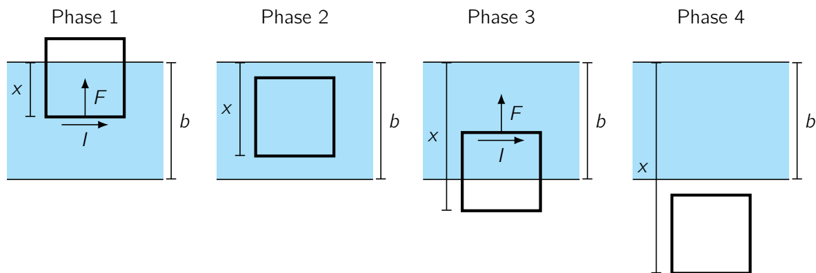
Abb. 8. Skizzen der vier Phasen des Falls der Leiterschleife.
