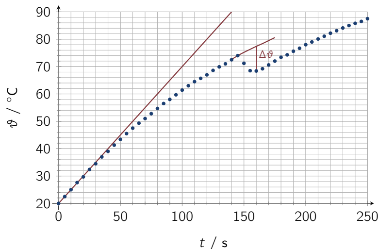
Abb. 10. Temperatur \vartheta im Wasserkocher in Abhängigkeit von der Heizzeit t mit konstruierten Größen für die Lösung.
