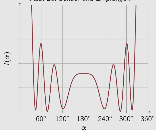
Abb. 21. Intensitätsverteilung in relativen Einheiten.
