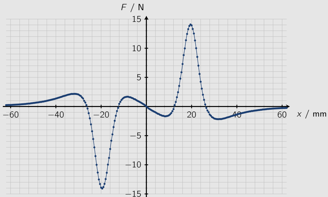
Abb. 6. Graph der Kraft auf den Stabmagneten in Abhängigkeit von der Position x .
