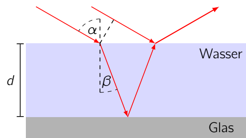
Abb. 19. Skizze zur Interferenzentstehung mit überhöhten Einfallswinkeln.
