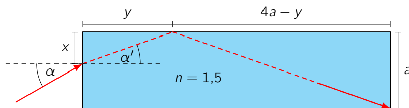
Abb. 14. Vollständige Skizze des Strahlenverlaufs im Glasquader in der Seitenansicht
