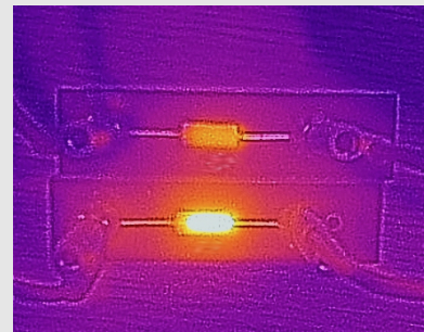
Abb. 11. Infrarotaufnahme der Widerstände.
