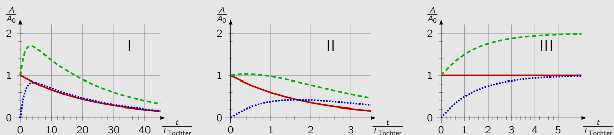
Abb. 22. Zeitliche Verläufe der Aktivitäten A sowohl des Mutternuklids als auch des Tochternuklids sowie der Gesamtaktivität der Präparate relativ zur Anfangsaktivität des Mutternuklids. Die Zeitachsen sind nach Vielfachen der Halbwertszeiten T_{\text{Tochter}} des jeweiligen Tochternuklids skaliert.
