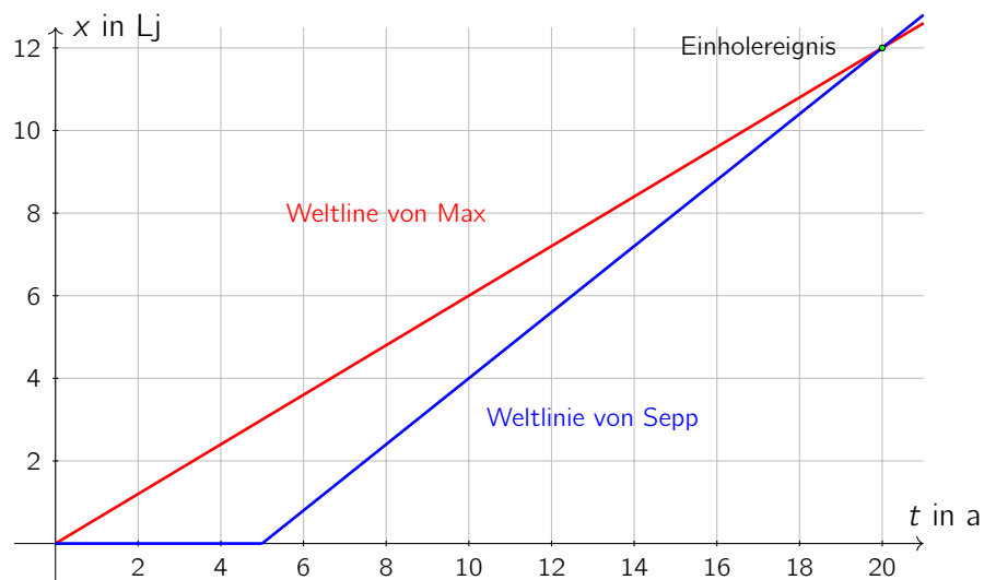
Abb. 24. Weltlinien der Zwillinge aus Sicht der Erde (quantitative Darstellung).
