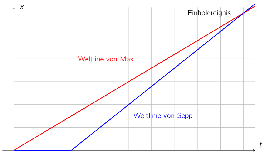
Abb. 23. Weltlinien der Zwillinge aus Sicht der Erde (qualitative Darstellung).
