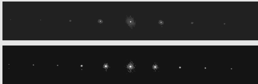
Abb. 17. Interferenzmuster auf dem Schirm für eine Wellenlänge von 650 nm (oben) und eine zweite unbekannte Wellenlänge (unten). Die Bilder zeigen den gleichen Ausschnitt des Schirms.
