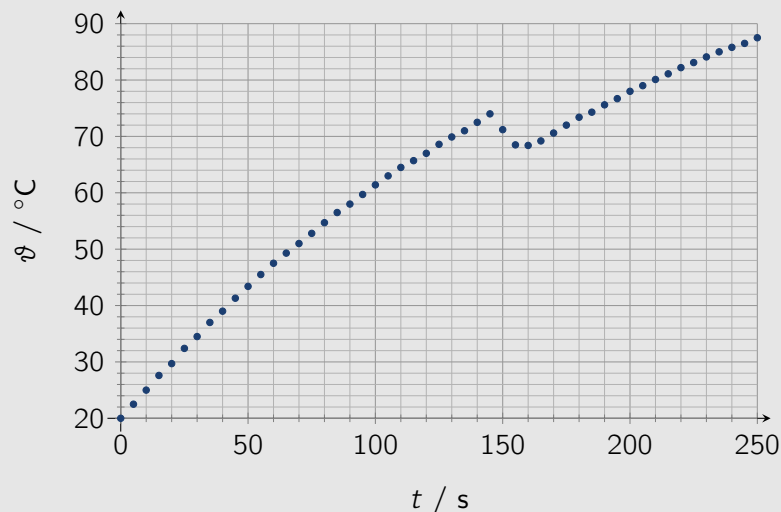
Abb. 9. Temperatur \vartheta im Wasserkocher in Abhängigkeit von der Heizzeit t .
