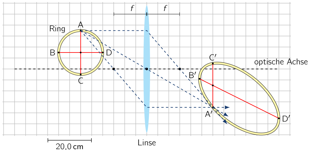
Abb. 15. Lösungsskizze zur Abbildung des Rings. Die Dicke des Rings wurde bei der Abbildung nicht berücksichtigt.
